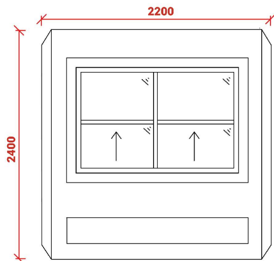
Elevación Sur
