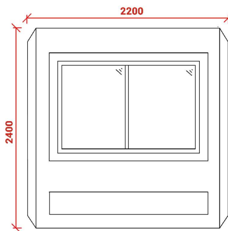
Elevación Norte
